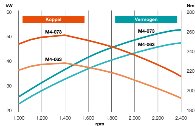
Vermogen en koppel
